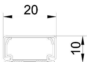
Canaleta 20x10
