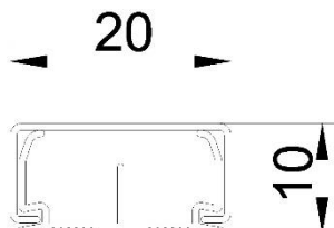
Canaleta 20x10
