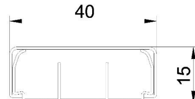
Canaleta 40x15
